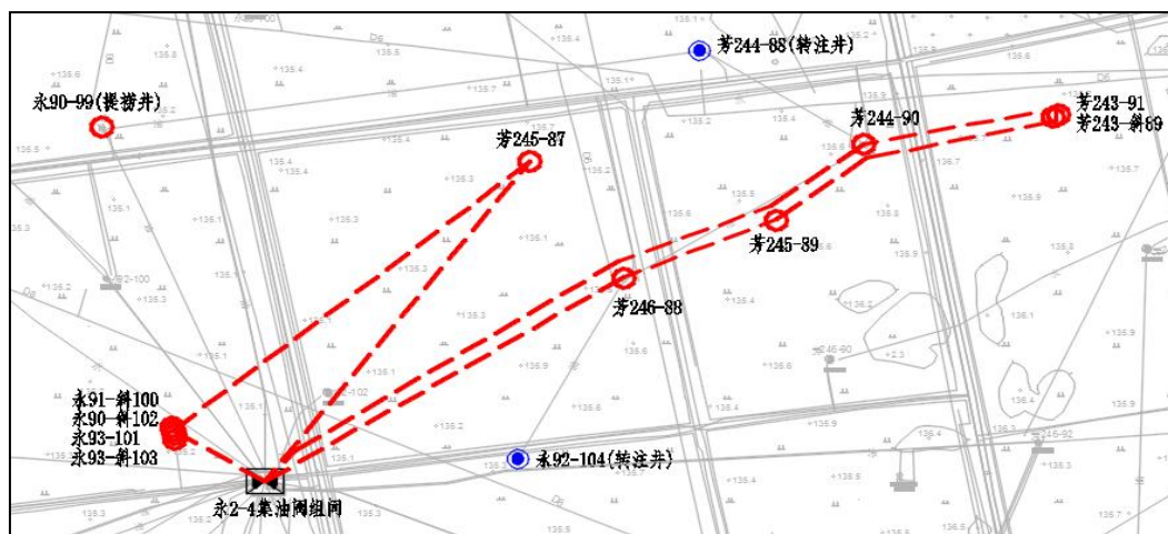
图 3-1-5 永 2-4 集油阀组间 2 环、5 环管道优化后管道走向示意图 ( ———— 现有管线走向, - - - - - 改造后管线走向)
