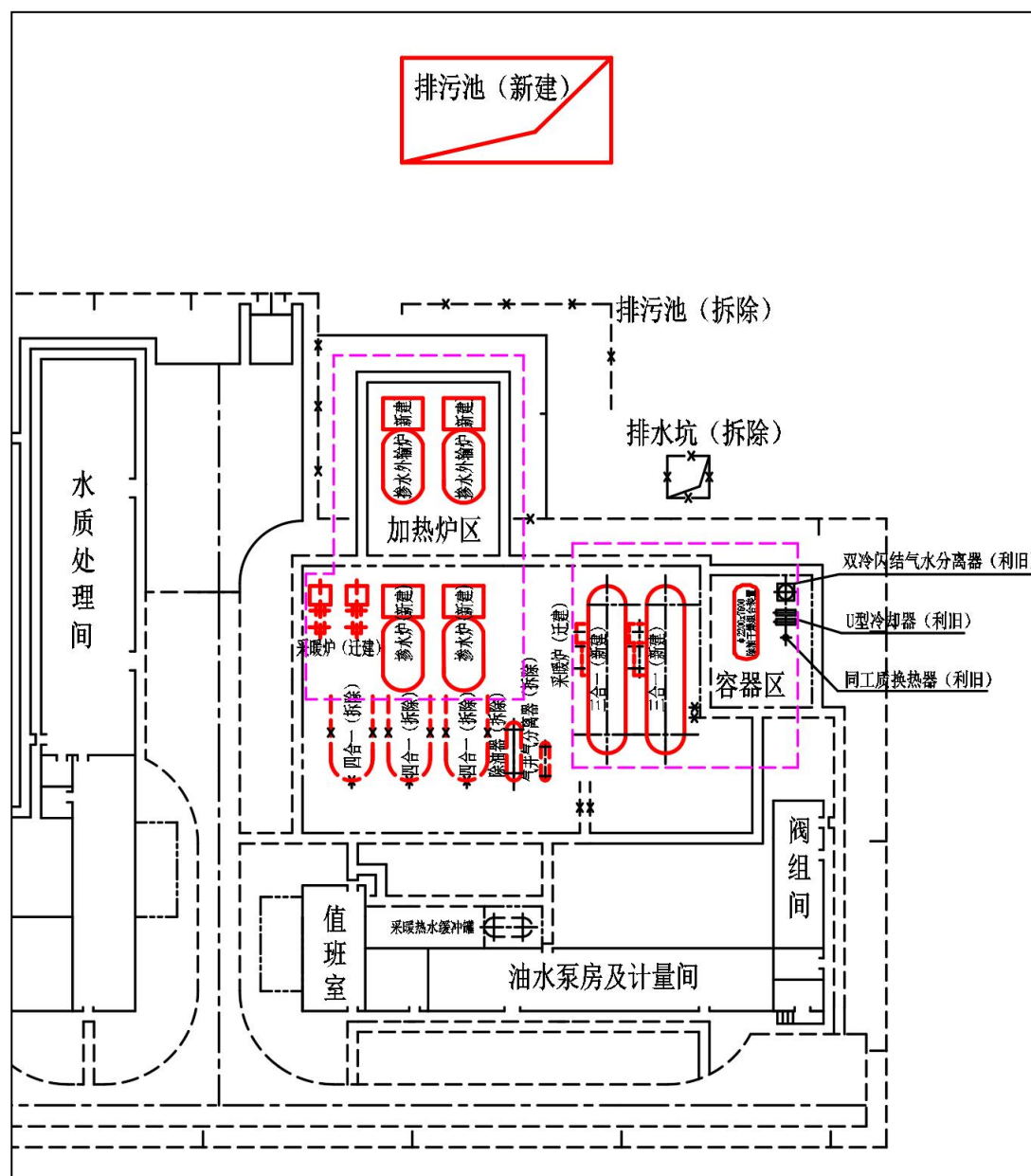
图 3-1-1 平面布置图
