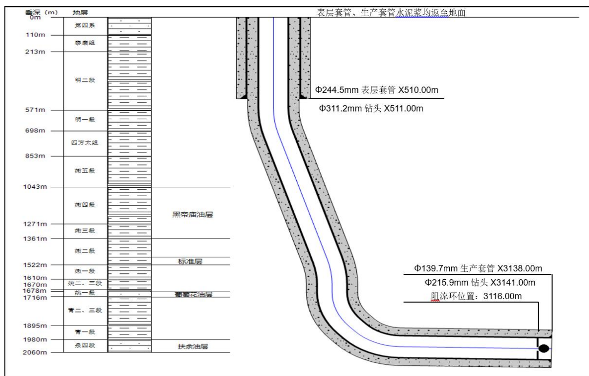
图 3.6-1 井身结构示意图
