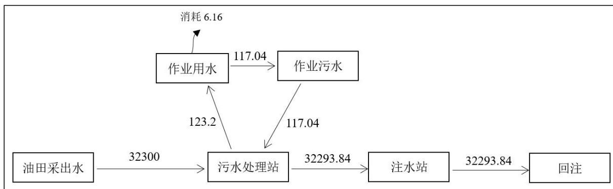
图 3.6-11 运营期水平衡图 (单位 \text{m}^3/\text{a} )
