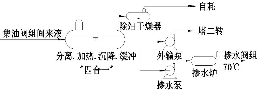
图 3.11-1 龙一转油站工艺流程图
