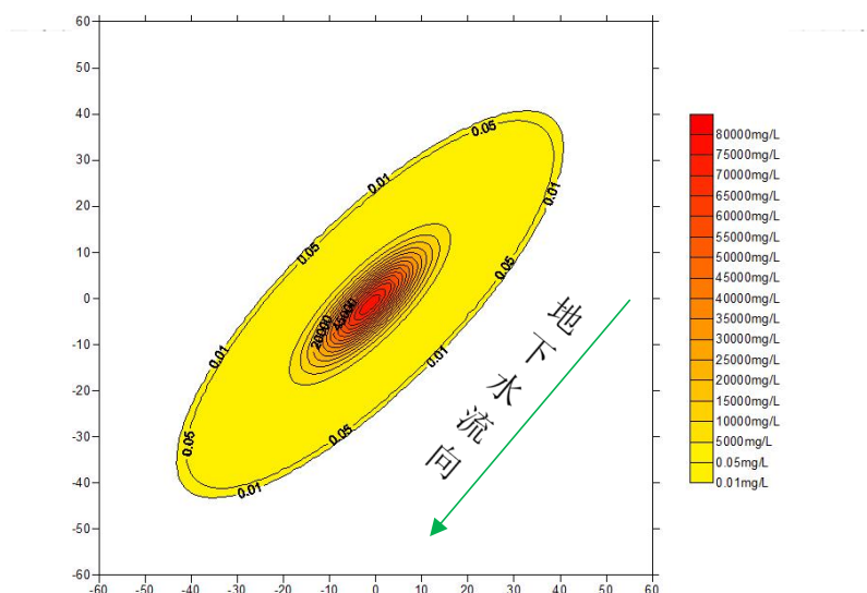
图 5.3-1 油基钻井液泄漏后 100 天污染物浓度分布图（污染源点：0，0）
