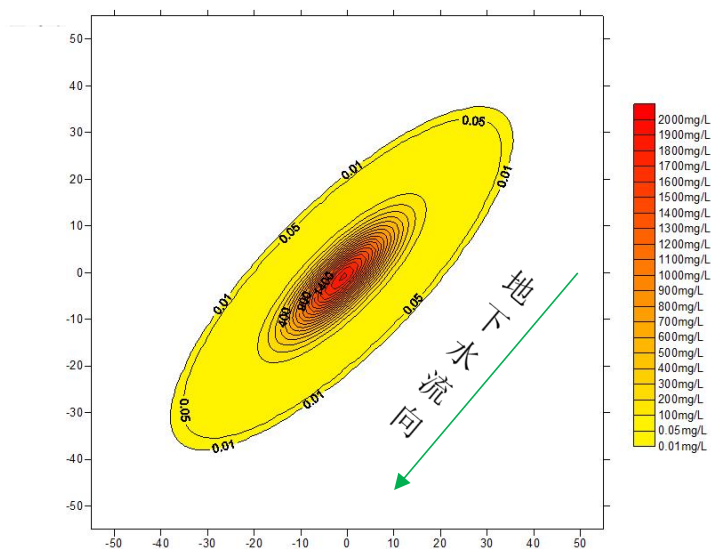
图 5.3-4 集油管道泄漏后 100 天污染物浓度分布图（污染源点：0，0）
