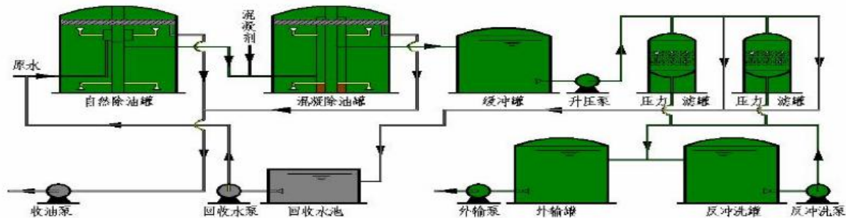
图3.11-2 龙一联合油污水处理站工艺流程
