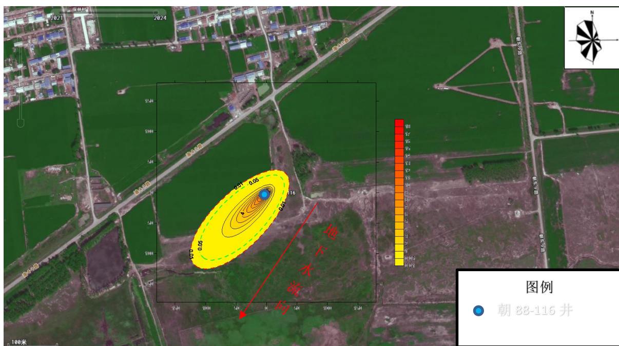
图 5.3-16 注水井套管泄漏 5475 天石油类污染扩散平面图（污染源点：0，0）
