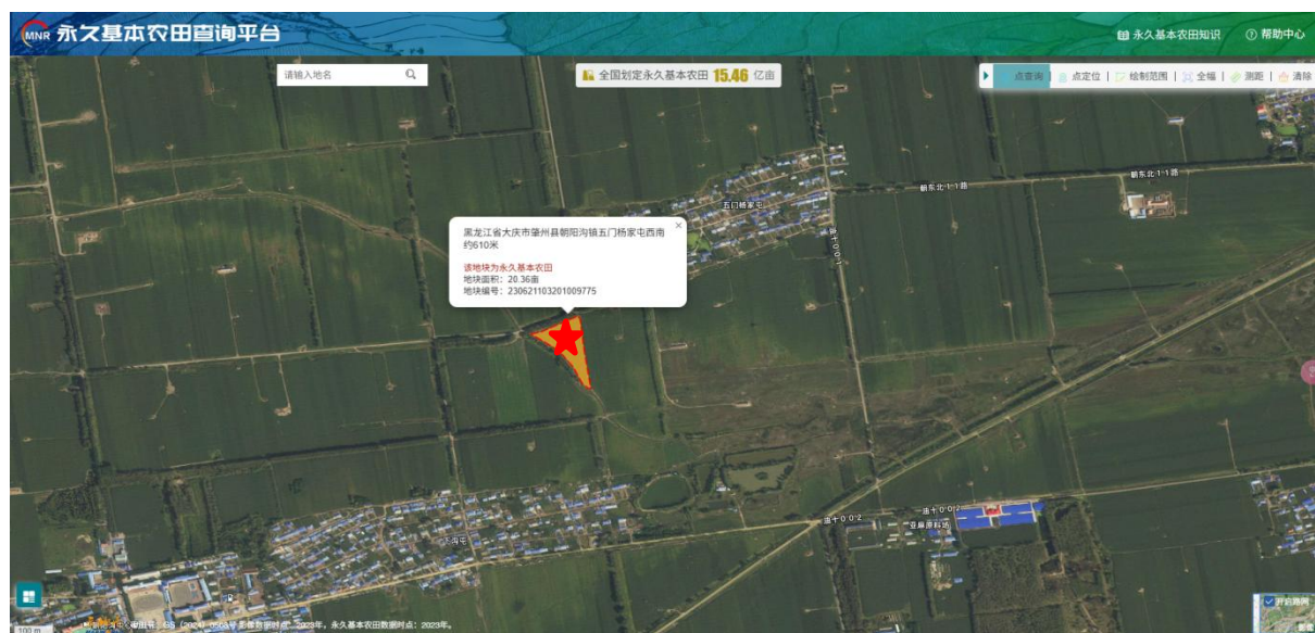
图 1.4-5 拟建朝 85-斜 99 井场与永久基本农田位置关系
