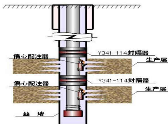
图 5.3-14 全过程一体化分注管柱示意图
