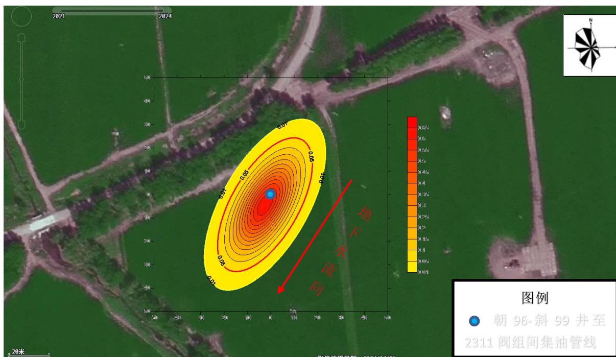
图 5.3-8 集油管道全管径泄漏后 1000 天污染物浓度分布图（污染源点：0，0）
