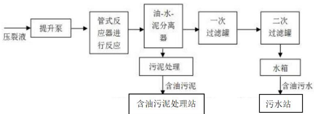
图 3.12-5 朝一联压裂返排液无害化处理站工艺流程图
