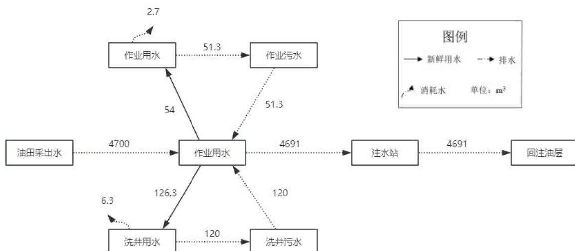
图 3.6-7 运营期水平衡图（单位 \text{m}^3/\text{a} ）
