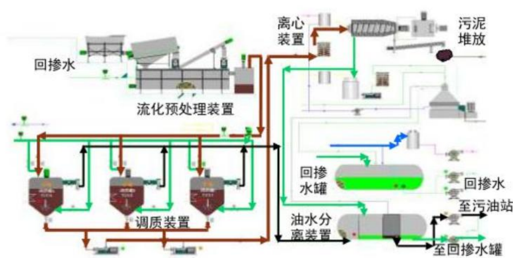
图 3.12-3 朝一联含油污泥处理站工艺流程图
