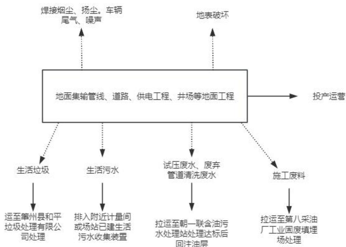
图 3.13-5 本项目地面工程施工期产污环节图
