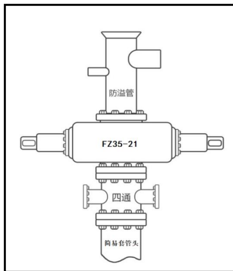
图 3.6-3 二开井口装置示意图
