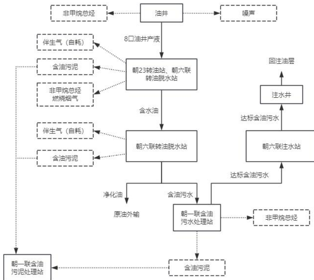
图 3.13-5 运营期正常工况工艺流程及产污示意图
