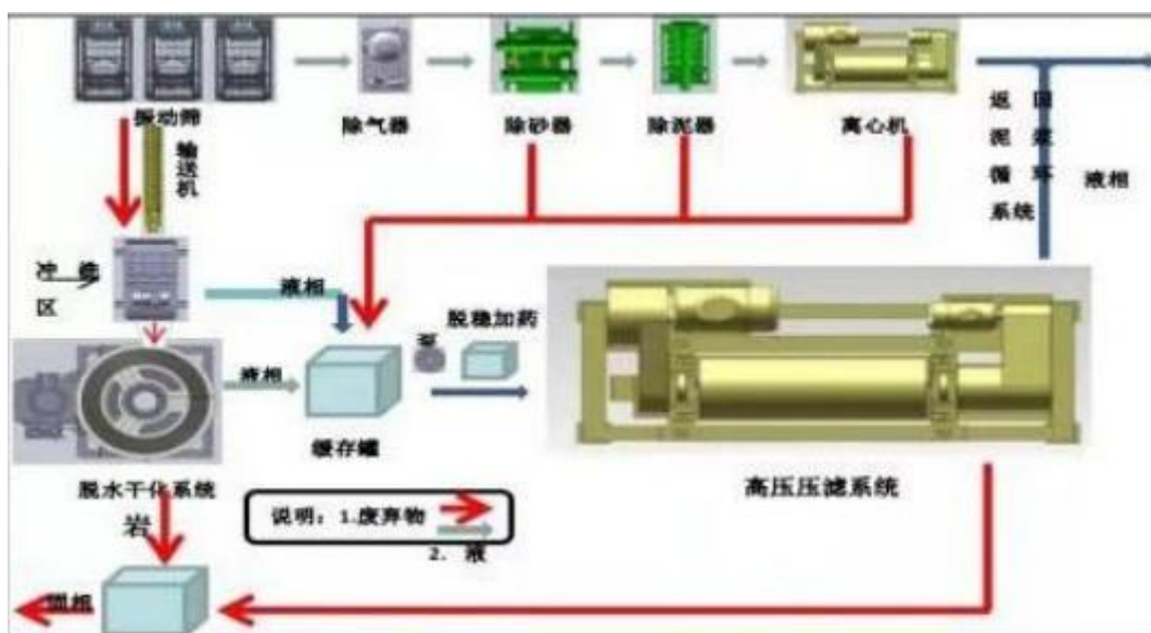
图 3.12-7 黑龙江龙之润环保工程有限公司工艺流程图
