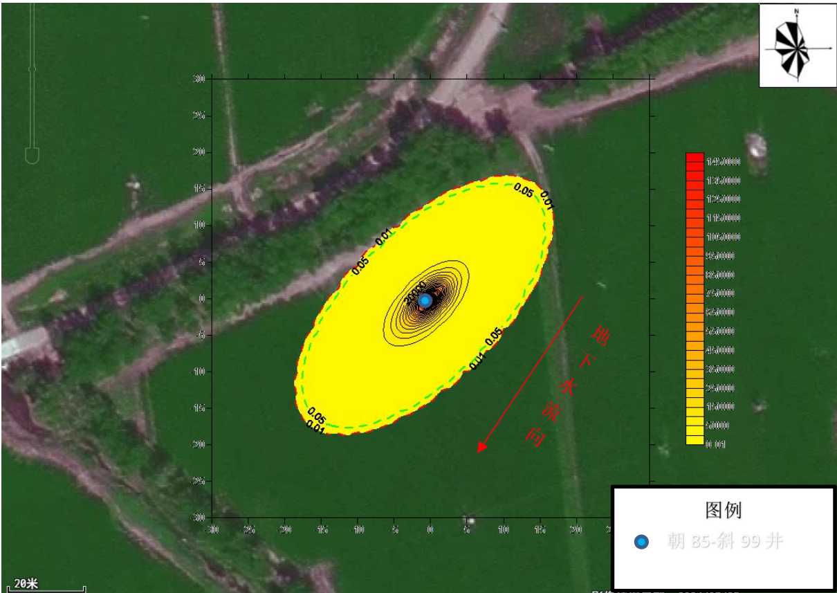
图 5.3-10 油井套管泄漏 100 天石油类污染扩散平面图（污染源点：0，0）
