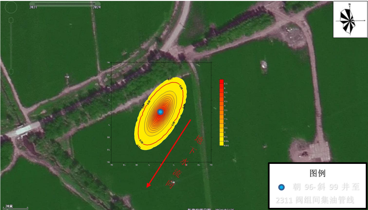
图 5.3-7 集油管道全管径泄漏后 100 天污染物浓度分布图（污染源点：0，0）
