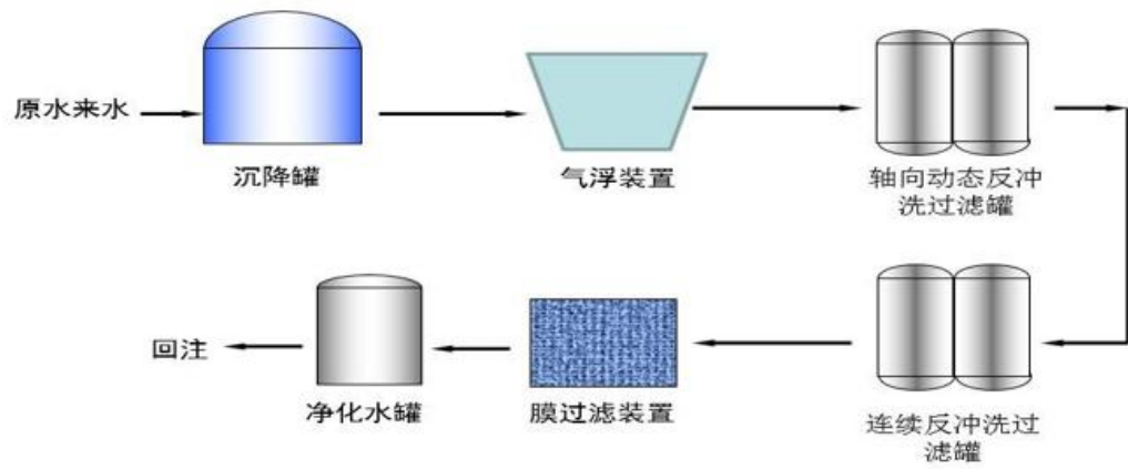
图 3.12-2 朝一联含油污水处理站工艺流程
