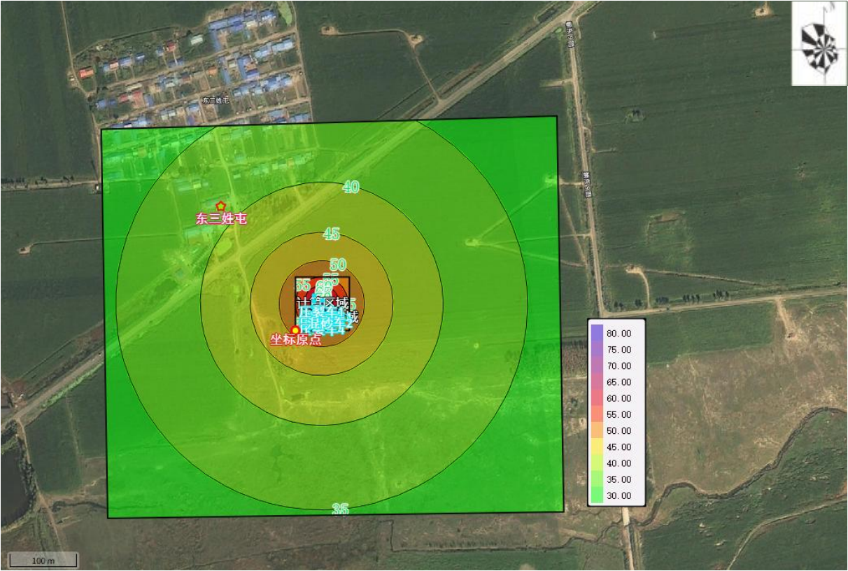
图 5.4-2 压裂施工期井场噪声预测图
