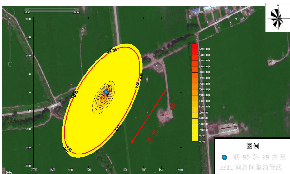
图 5.3-6 集油管道 10%管径泄漏后 5475d 污染物浓度分布图 (污染源点: 0, 0)
