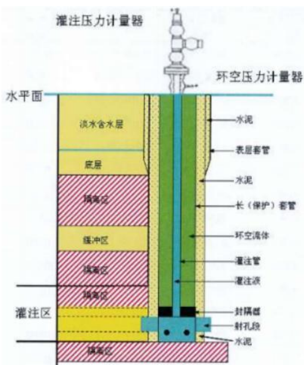
图 5.3-13 注水井井身结构示意图
