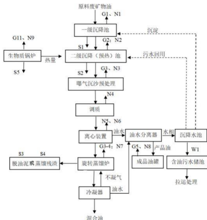
图 3.12-6 大庆市顺和环保科技有限公司工艺流程图
