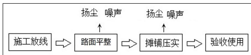
图 3.13-4 通井路施工流程图
