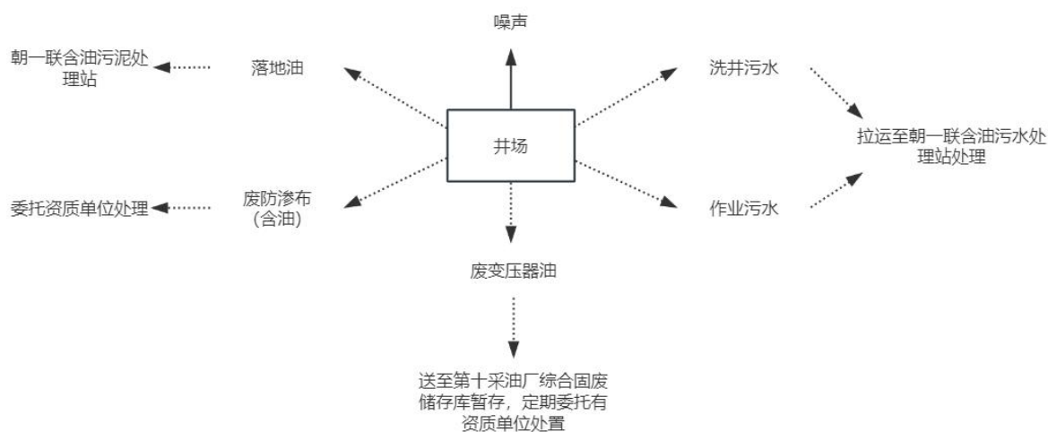
图 3.13-6 运营期非正常工况工艺流程及产污示意图
