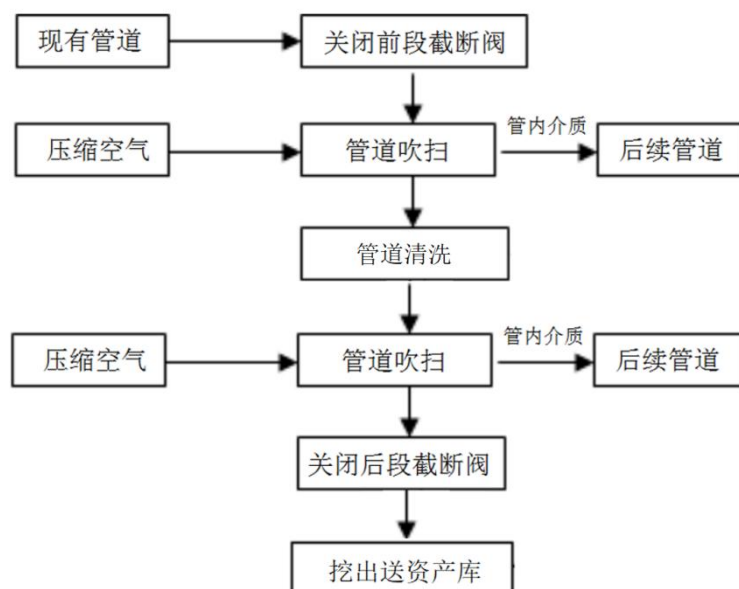
图 3.8-1 原有管道处理流程图
