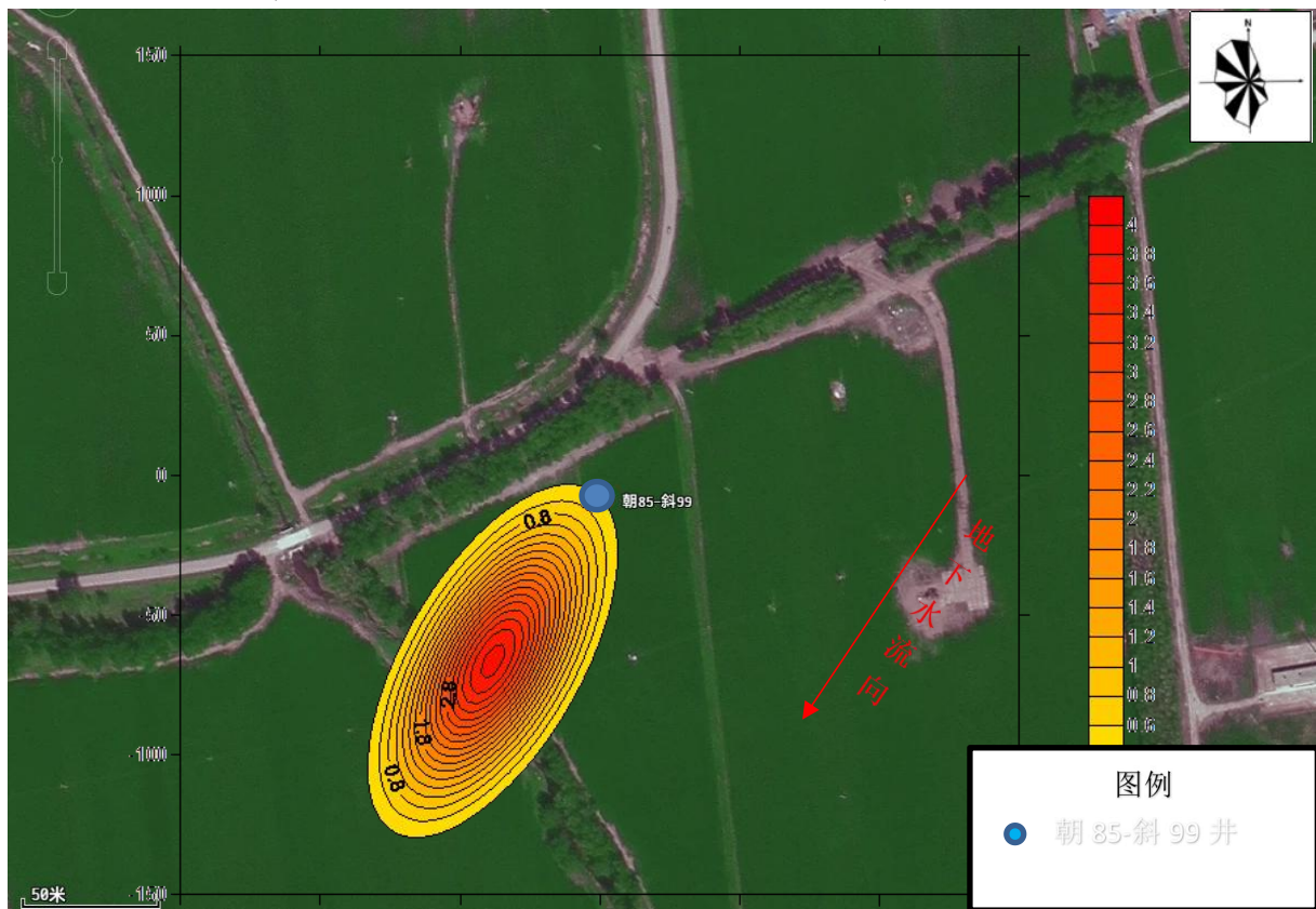
图 5.3-3 水基钻井液泄漏后 5475 天污染物浓度分布图（污染源点：0，0）
