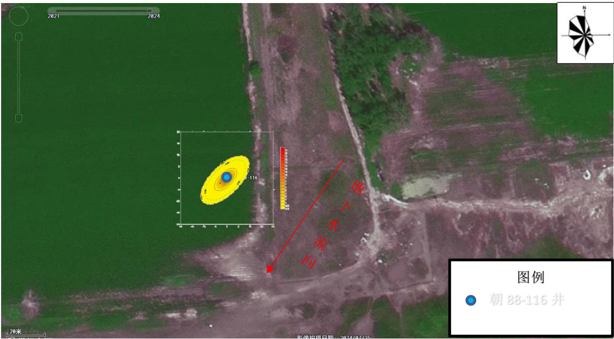
图 5.3-14 注水井套管泄漏 100 天石油类污染扩散平面图（污染源点：0，0）
