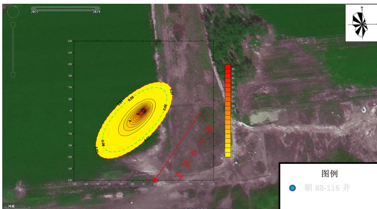
图 5.3-15 注水井套管泄漏 1000 天石油类污染扩散平面图（污染源点：0，0）
