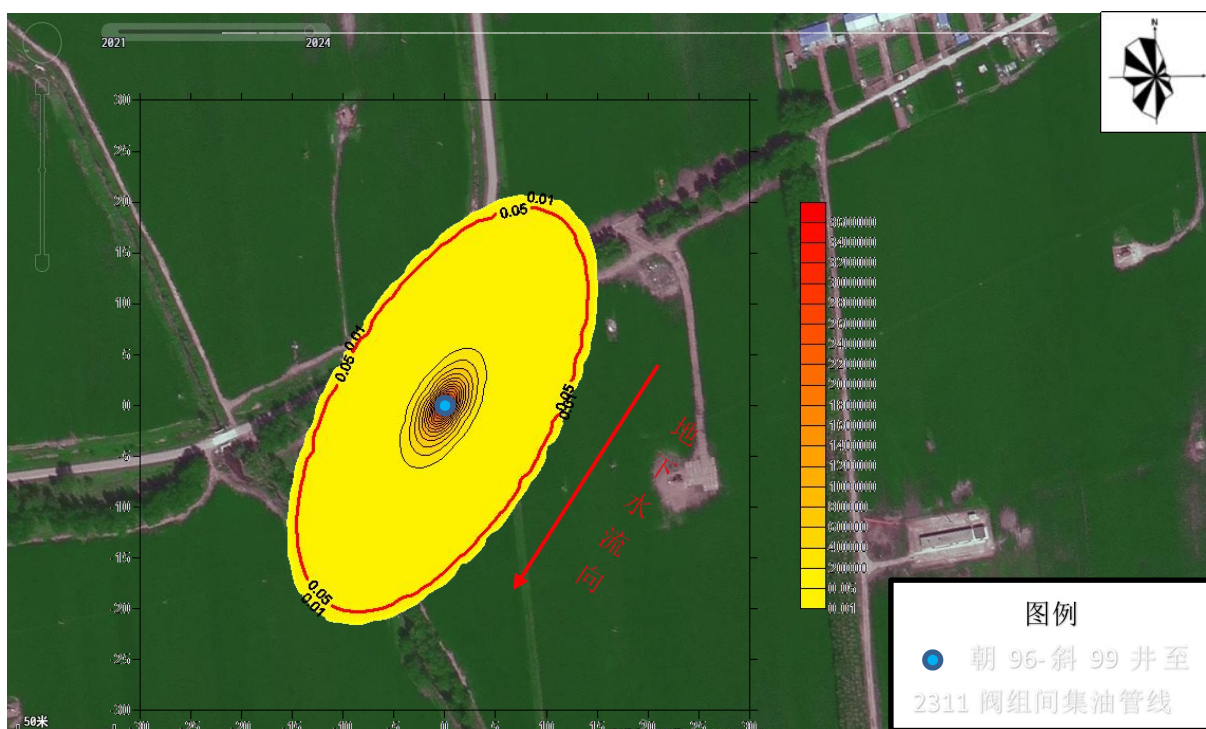
图 5.3-4 集油管道 10%管径泄漏后 100d 污染物浓度分布图（污染源点：0，0）
