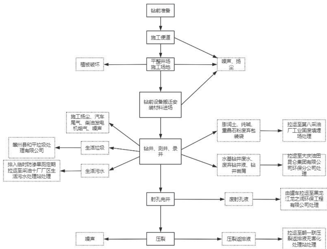
图 3.13-1 本项目钻井及储层改造工艺流程及产污环节图
