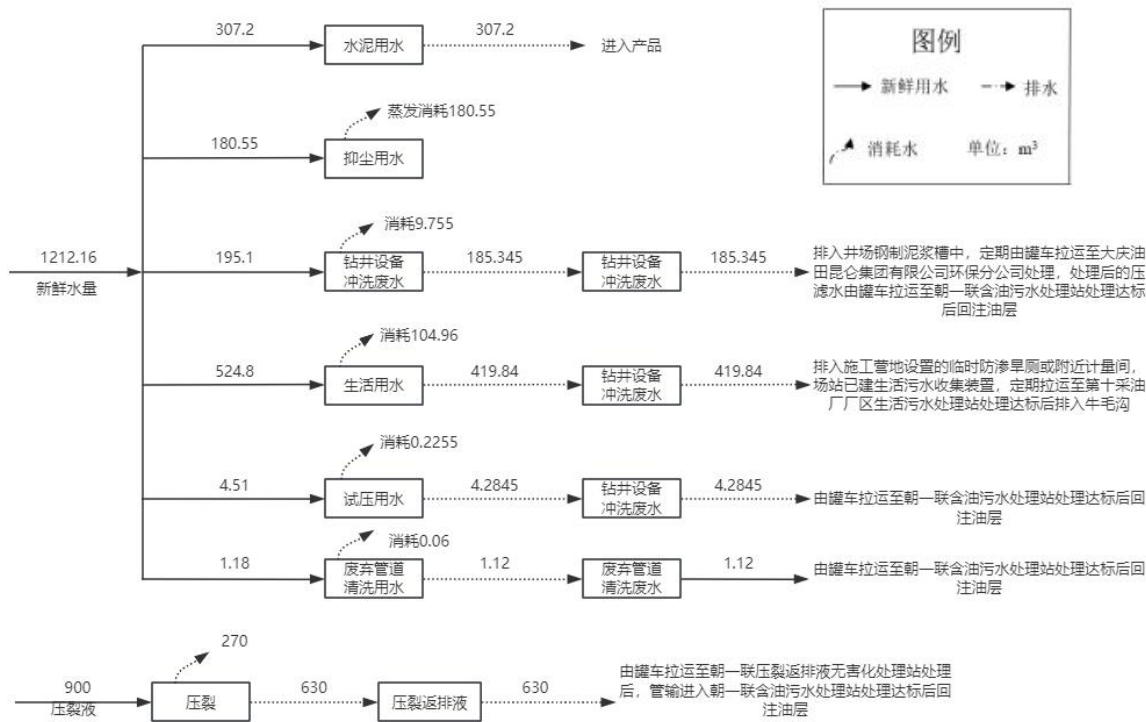
图 3.6-6 施工期水平衡图 (单位: m³)
