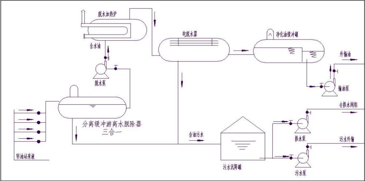
图 3.12-1 朝六联转油脱水站工艺流程图
