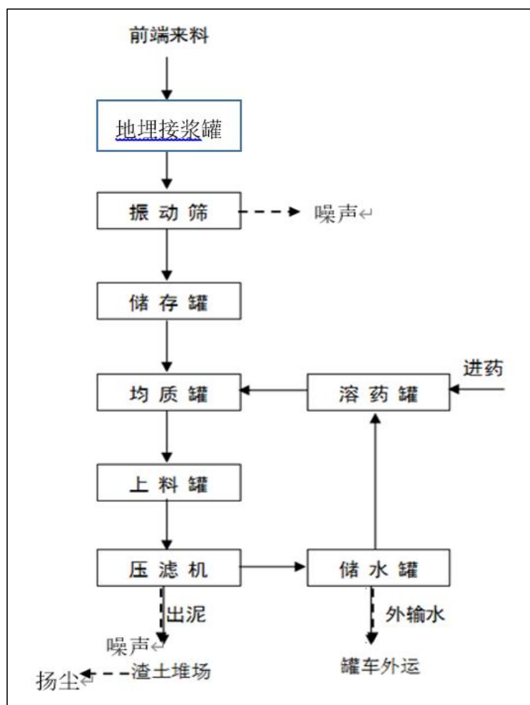
图 3.12-4 大庆油田昆仑集团有限公司环保分公司工艺流程图
