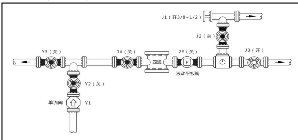
图 3.6-4 二开井口管汇示意图
