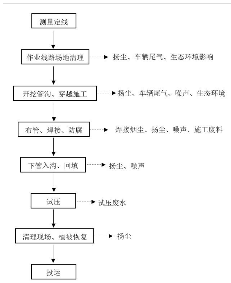
图 3.13-3 管线施工过程产污节点图
