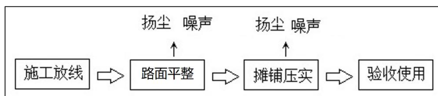
图 3.8-4 道路施工建设过程
