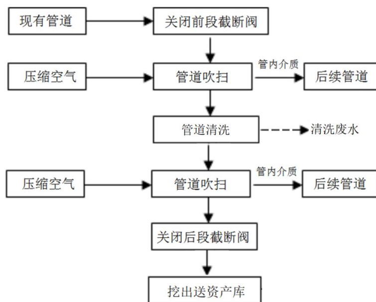
图 3.13-2 原有管道处理工艺流程图
