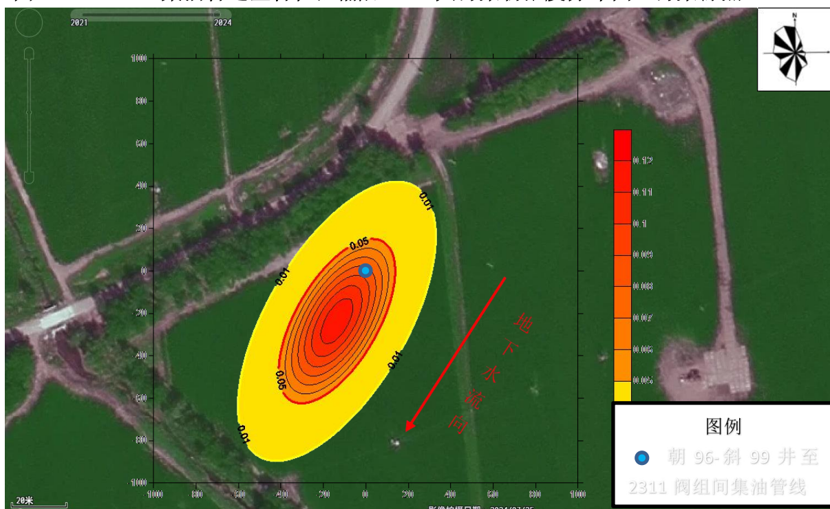
图 5.3-9 集油管道全管径泄漏后 5475 天污染物浓度分布图（污染源点：0，0）
