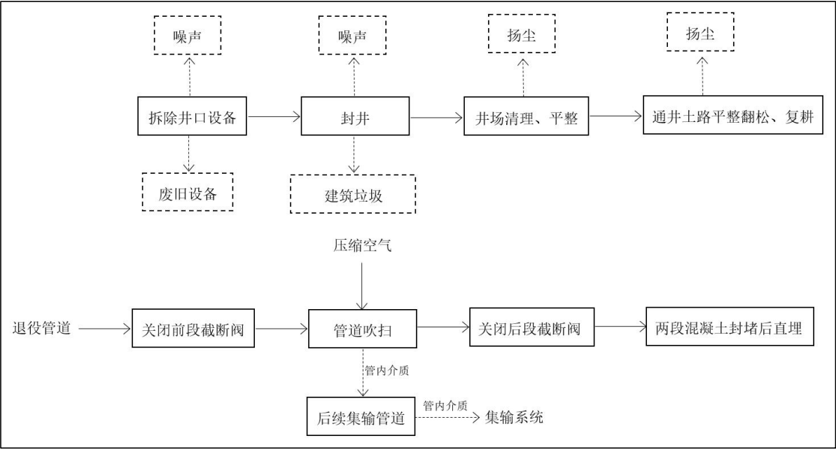
图 3.13-7 退役期工艺流程及主要产污节点图
