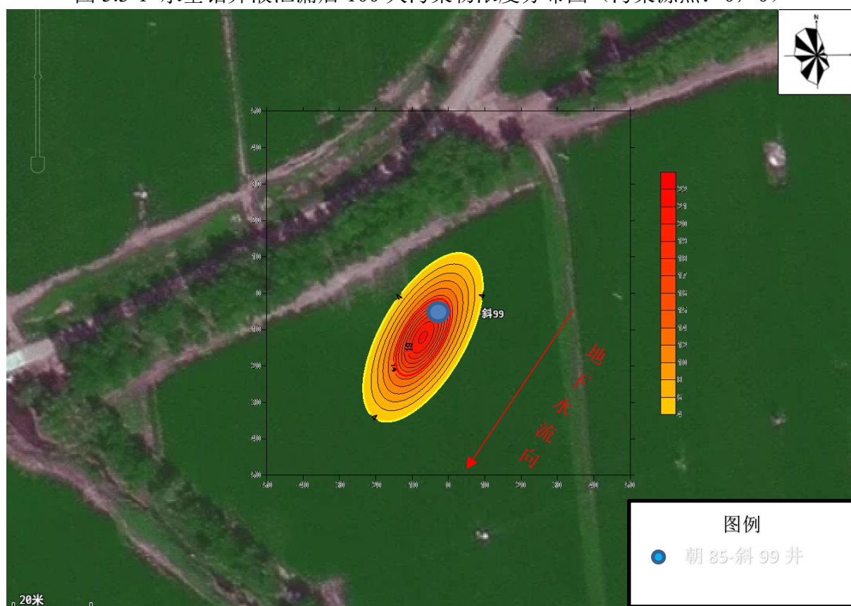
图 5.3-1 水基钻井液泄漏后 100 天污染物浓度分布图（污染源点：0，0）
