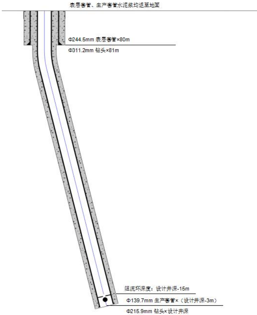
图 3.6-1 定向井井身结构示意图
