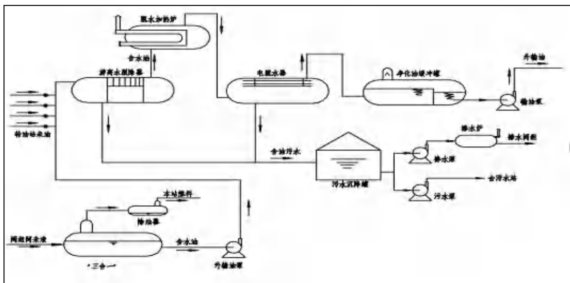
图 2.4-1 宋二联脱水站工艺流程图
