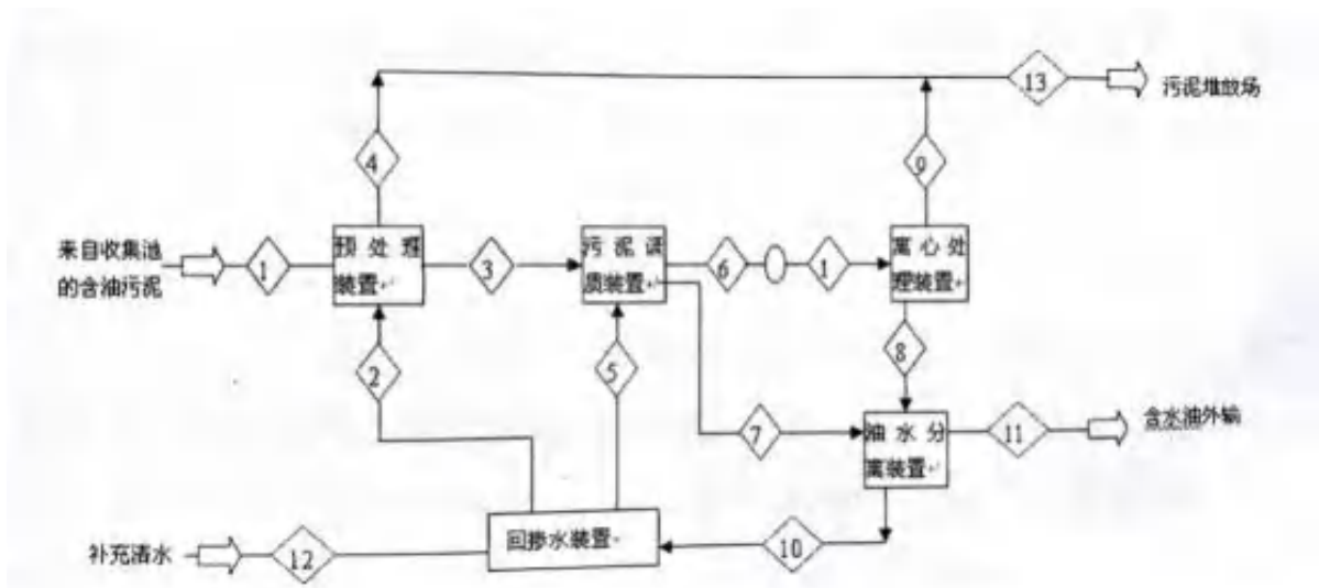
图 2.4-2 宋芳屯含油污泥处理站工艺流程图
