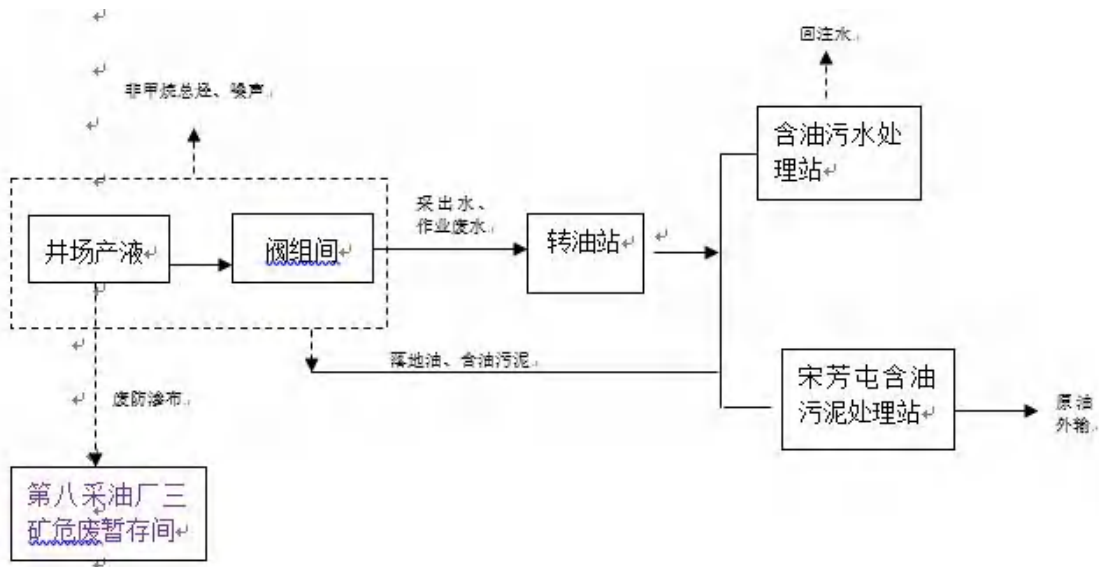
图 2.5-2 运行期工艺流程图
