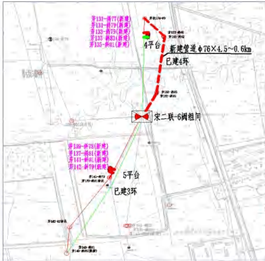
图 2.3-2 (3) 宋二联-6 阀组间集油管网布局
