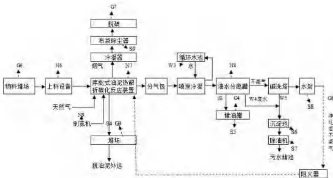
图 2.4-3 大庆市云泰石化产品有限公司序批式热解析装置生产工艺流程图
