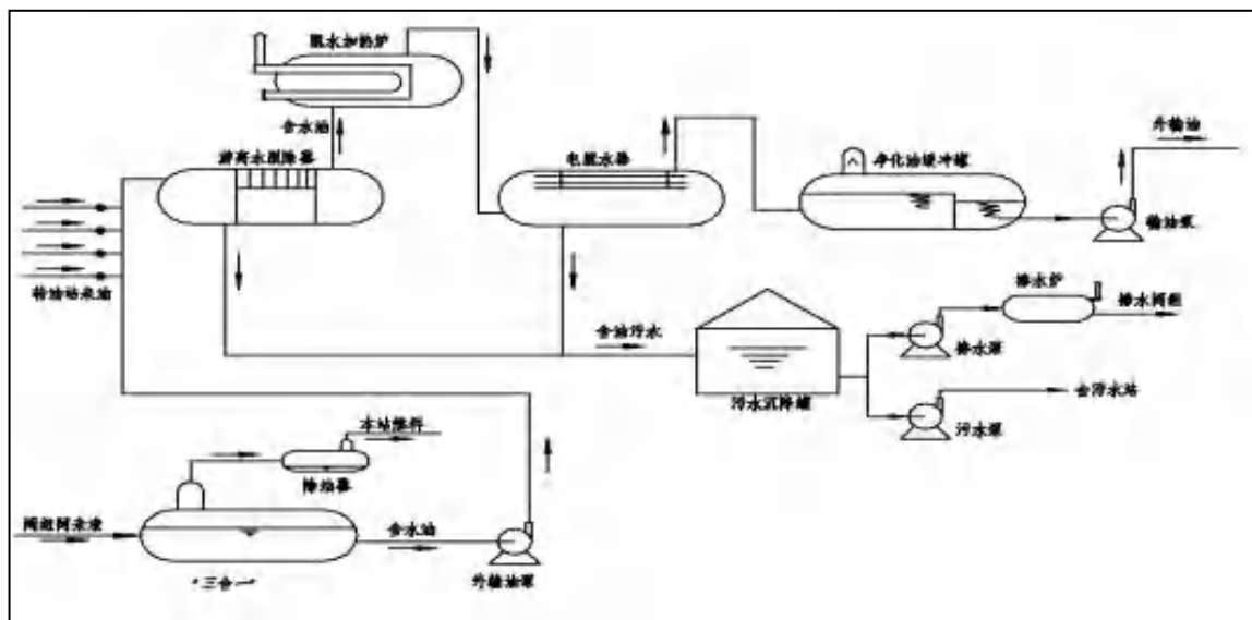
图 2.3-16 宋二联脱水站工艺流程图
