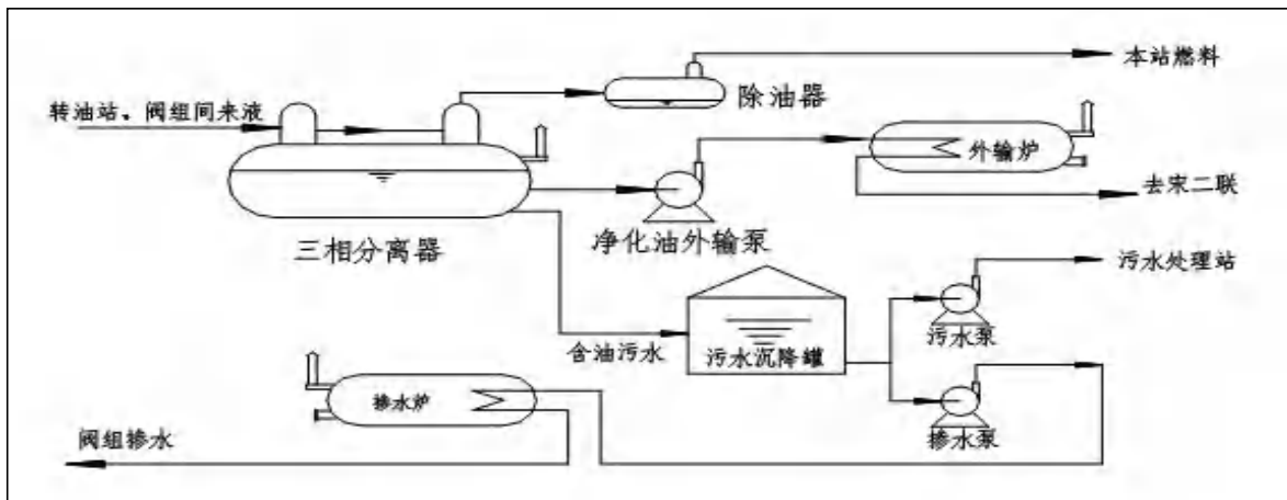
图 2.3-15 肇一联脱水站工艺流程图
