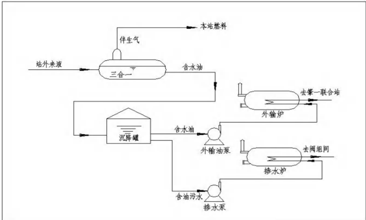
图 2.3-12 肇4转油站工艺流程
