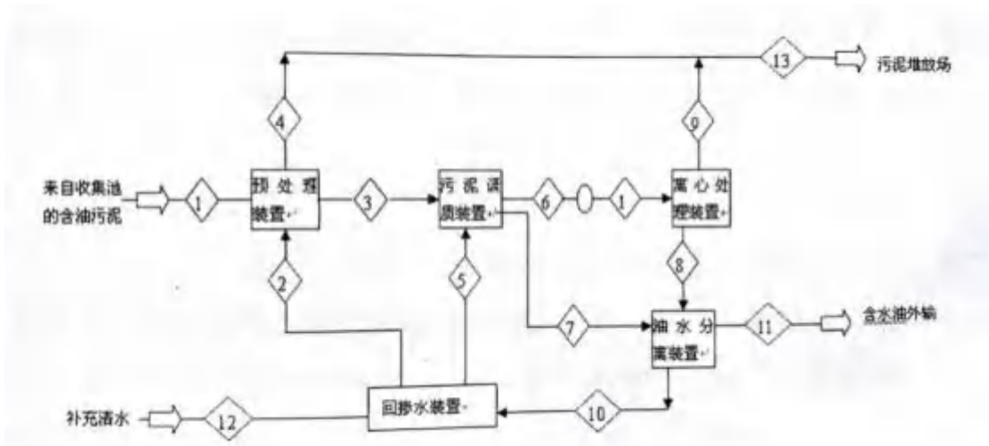
图 2.3-17 宋芳屯含油污泥处理站工艺流程图
