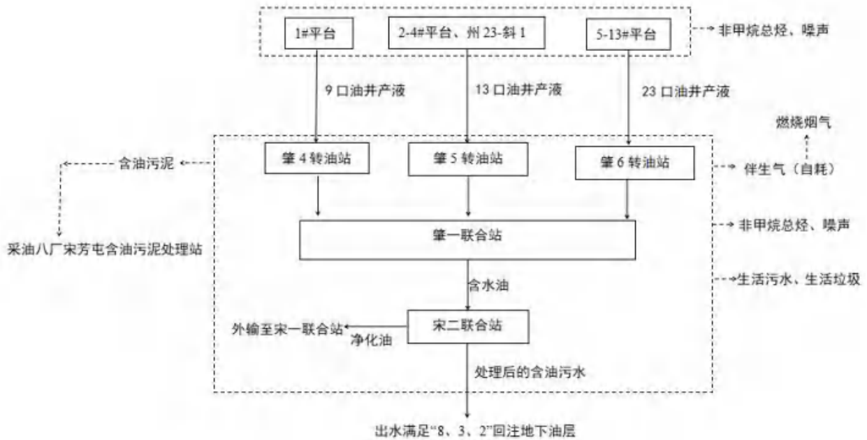
图 2.4-4 运行期工艺流程图
