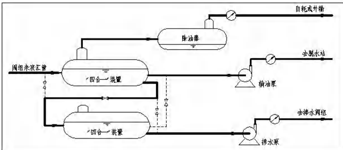
图 2.3-13 肇5转油站工艺流程
