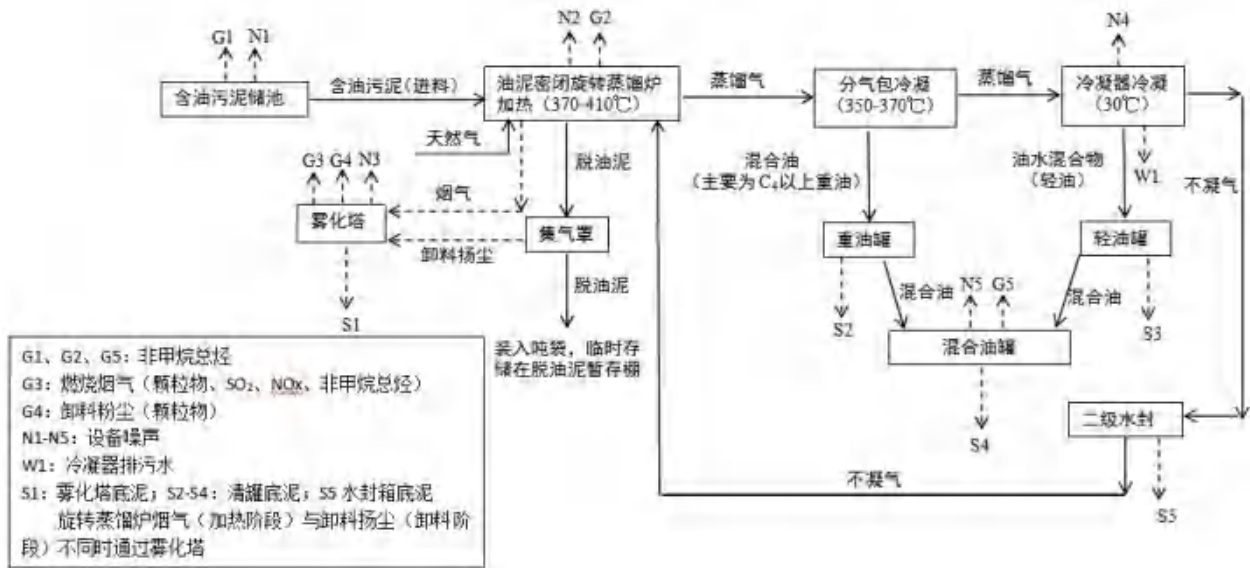
图 2.3-18 水务公司采油八厂含油污泥处理站工艺流程图
