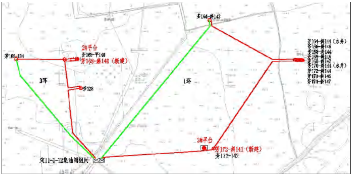
图2-4-6 (3) 2口井挂接宋II-3-12集油阀组间现有管线示意图
