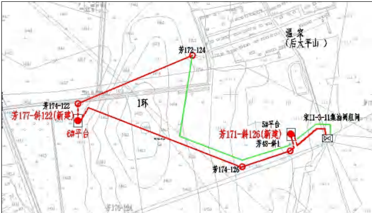
图2-4-6 (2) 2口井挂接宋II-3-11集油阀组间现有管线示意图
