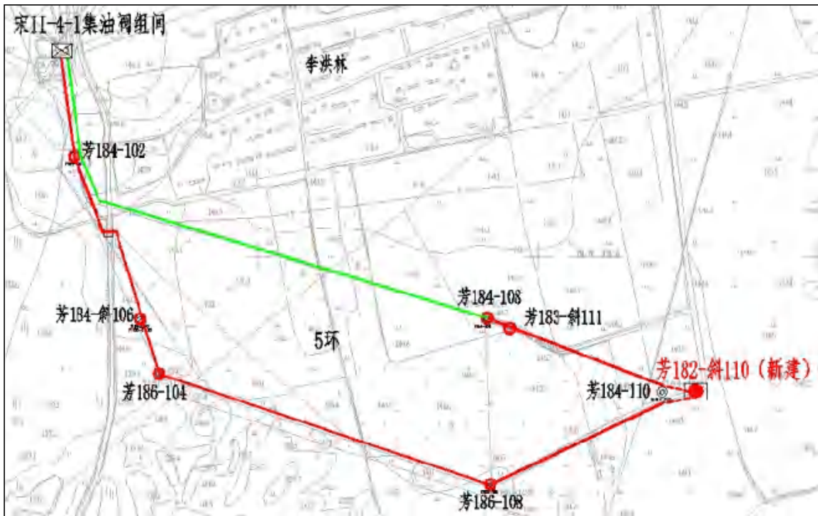
图2-4-6 (5) 1口井挂接宋II-4-1集油阀组间现有管线示意图
