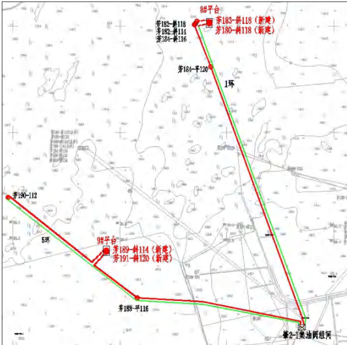
图 2-4-6 (7) 4 口井挂接肇 2-1 集油阀组间现有管线示意图
