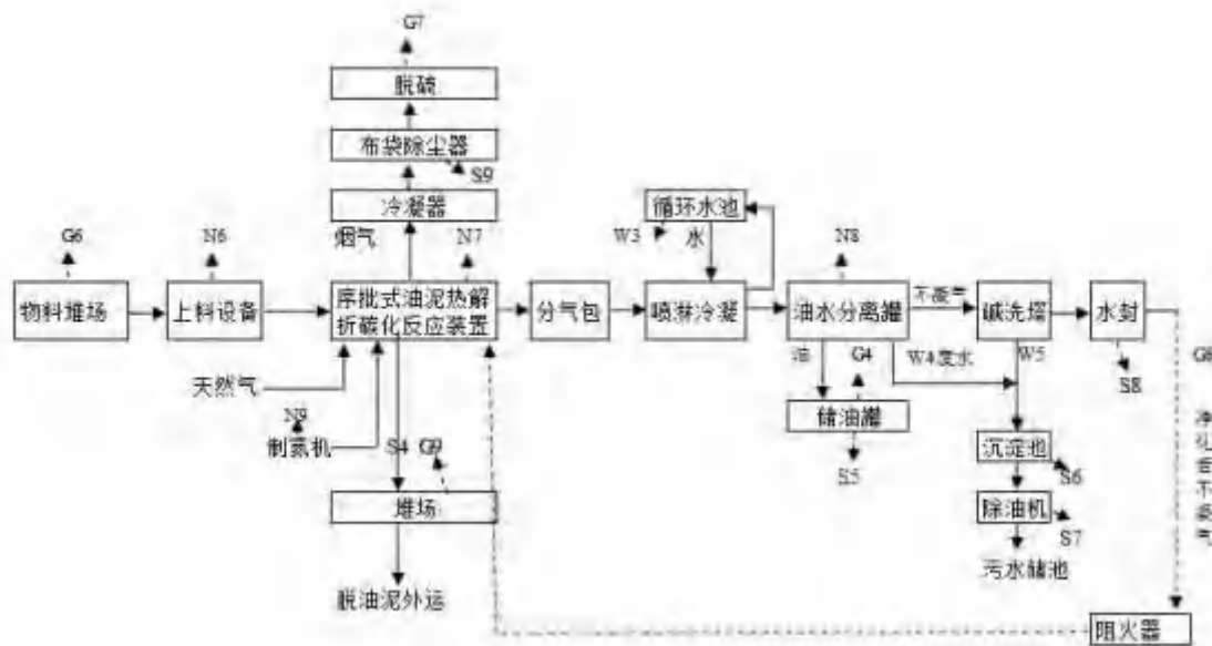
图 2.4-13 含油污泥处理工艺
