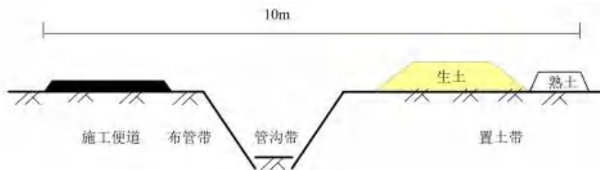
图 2.4-7 管道施工断面平面布置图
