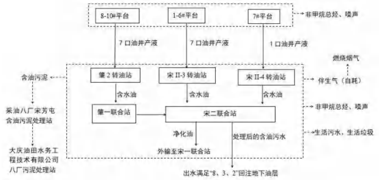
图 2.4-4 运行期工艺流程图
