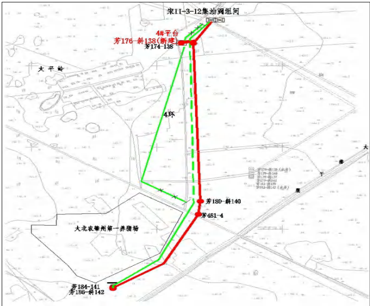
图2-4-6 (4) 1口井挂接宋II-3-12集油阀组间现有管线示意图
