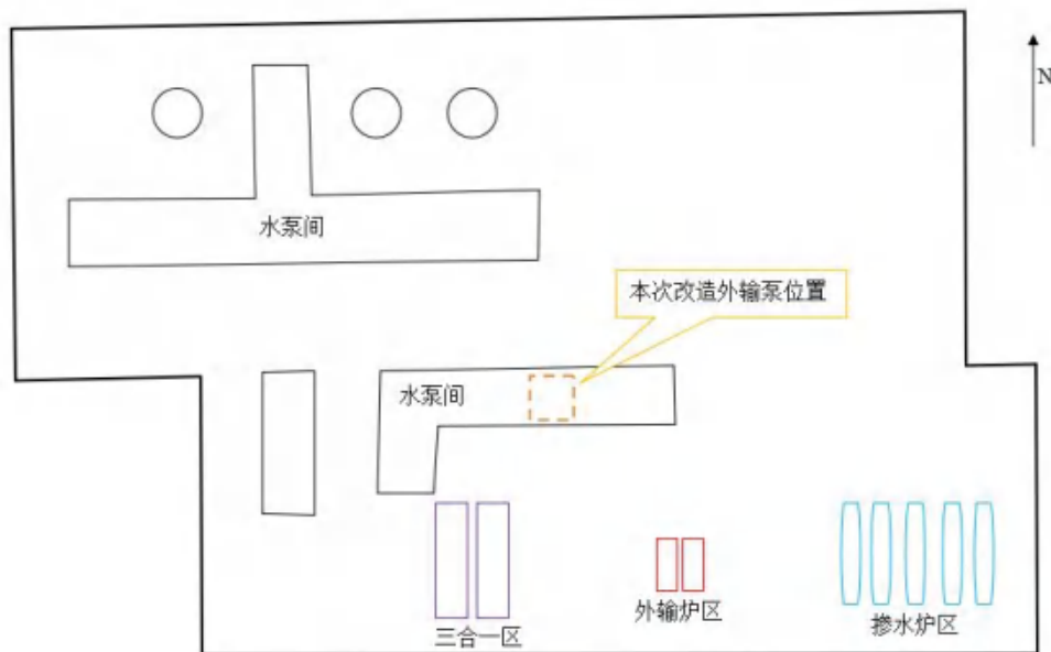
图 2-4-8 宋 II-3 转油站站内改造平面布置图
