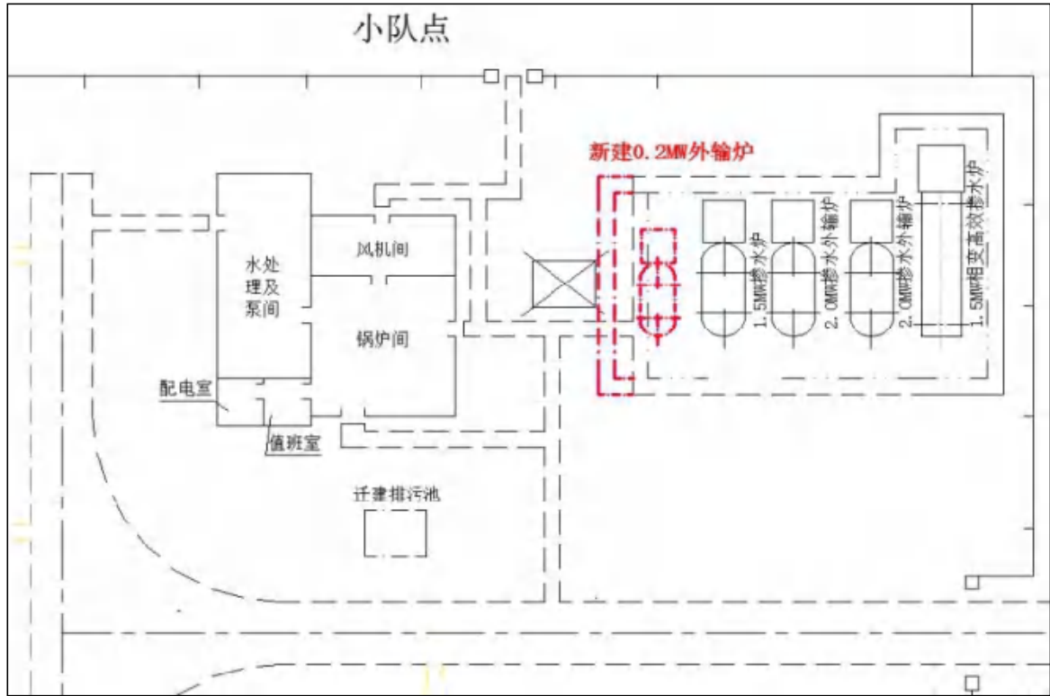
图2-4-9 肇2转油站站内改造平面布置图
