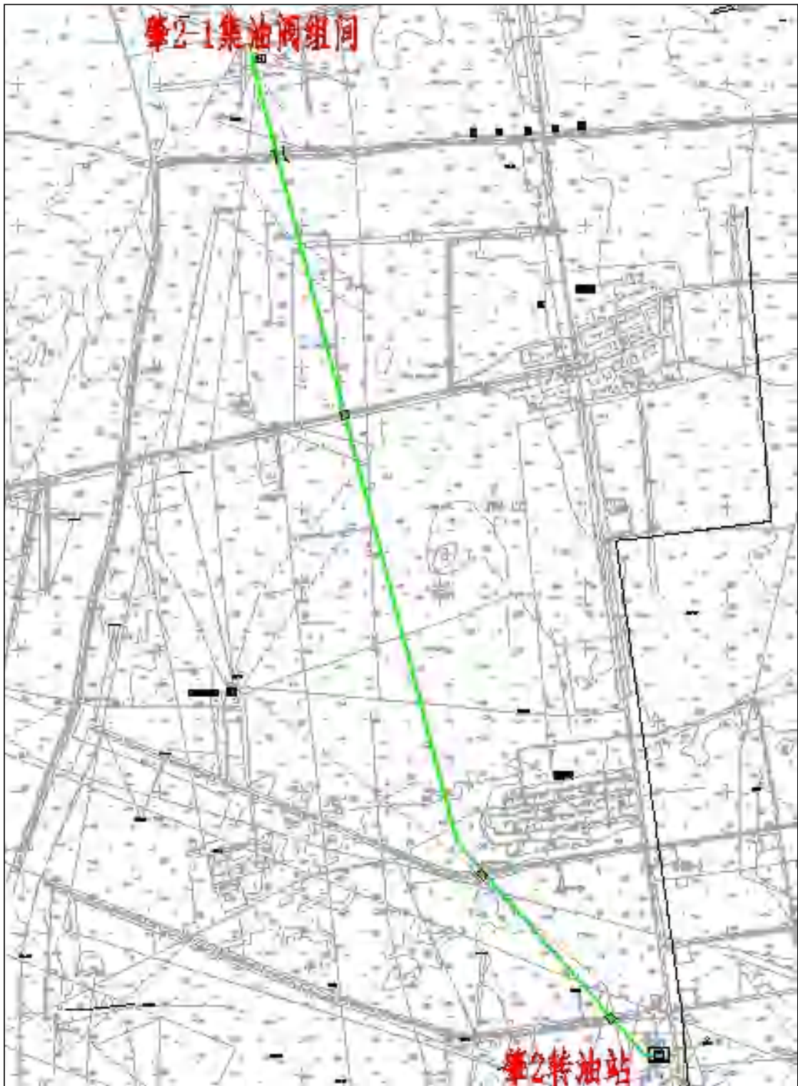
图 2-4-7（1） 更换肇 2-1 集油阀组间至肇 2 转油站间总掺水管线示意图
