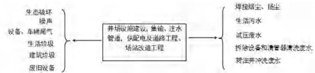
图 2.5-1 施工期工艺流程及产污节点图
